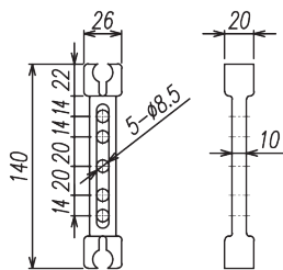
Separator : Ø8 (Aluminum)
