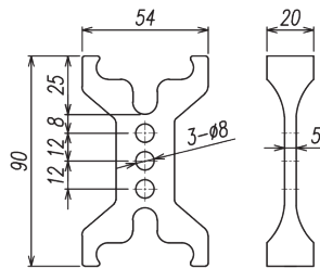
Separator : Ø8 (Aluminum)
