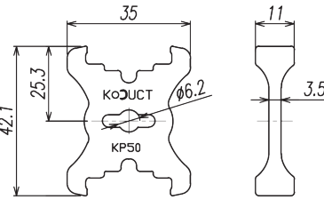
Separator : Ø6 (Aluminum)
