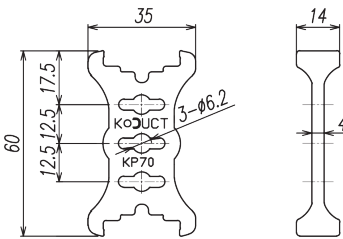
Separator : Ø6 (Aluminum)
